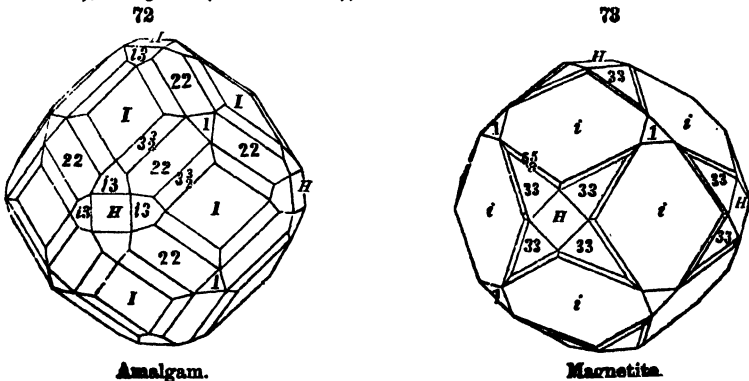
Amalgam.
